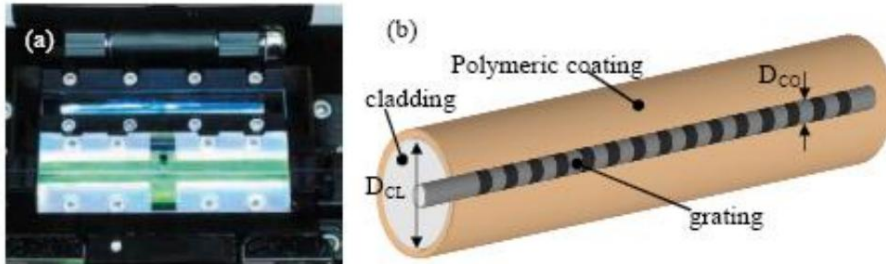
(a) Moules en quartz de la machine de revêtement (b) Schéma de principe du FBG uniformément revêtu.
